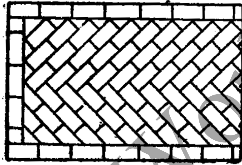
Fig 11.24 Zigzag Bond
